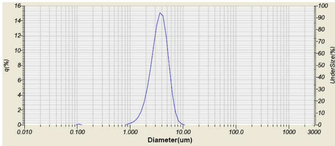
球形鋁粉粒徑分佈一例
